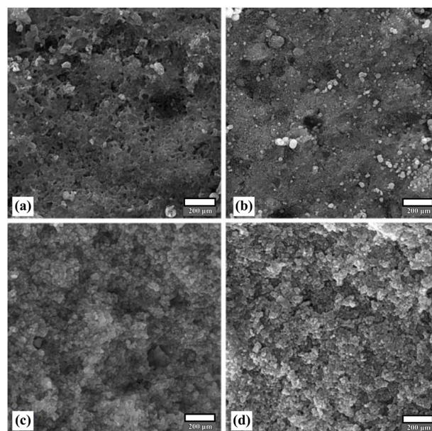
Fig. 4. SEM images of sintered specimens at 900 °C: (a) 0 wt. % \text{MgF}_2 ; (b) 5 wt. % \text{MgF}_2 ; (c) 7.5 wt. % \text{MgF}_2 ; (d) 10 wt. % \text{MgF}_2 .
